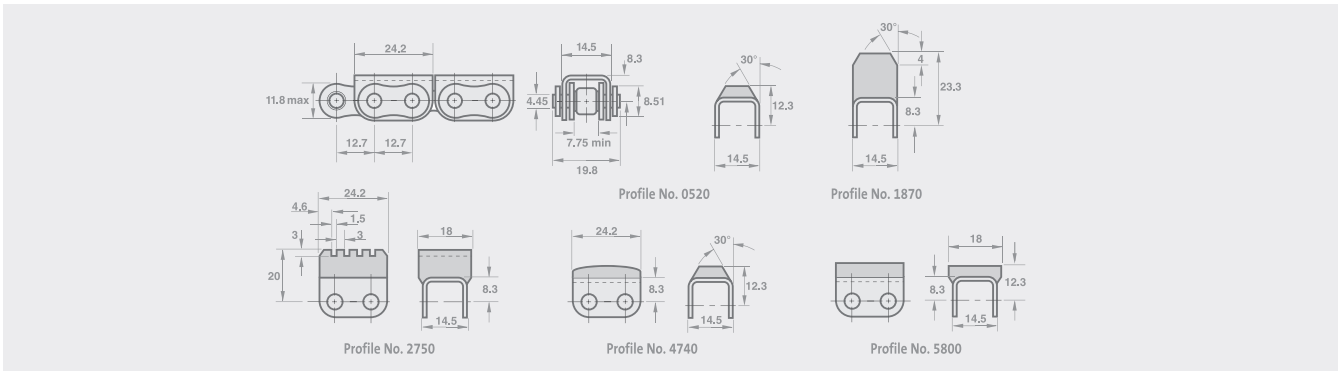
0.500英寸节距简单链条轮廓外形 0.500" pitch simple chain profiles
