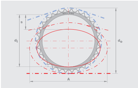
A的值包括与链轮之间的一个安全距离 Value A includes a safety distance to the sprockets
