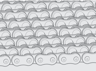
▲ 八排链 - 标准 Octuplex chain – Standard ANSI B29.1 ISO 606 A
